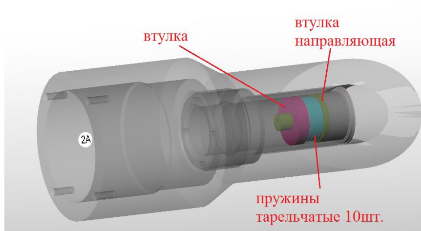
Рисунок 54 – пружины тарельчатые и штулки
