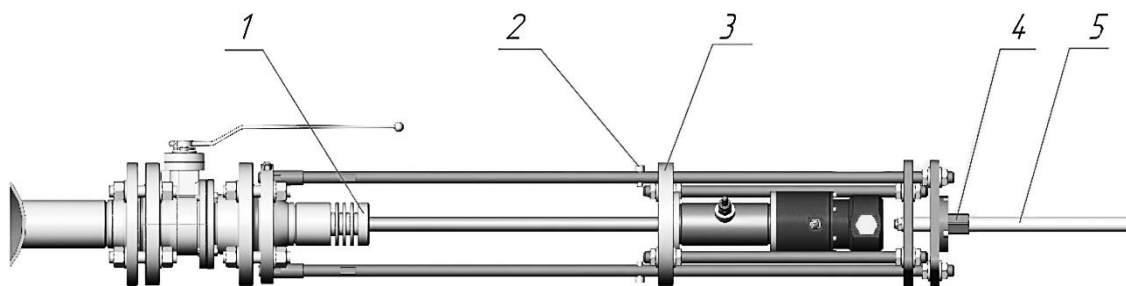
1 – Фланец установочный; 2 – Винт М8; 3 – Фланец плоский; 4 – Гайка; 5 — Винт ходовой.
