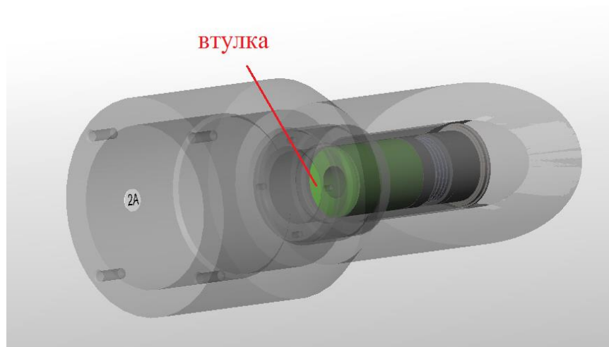
Рисунок 53 – штулка
