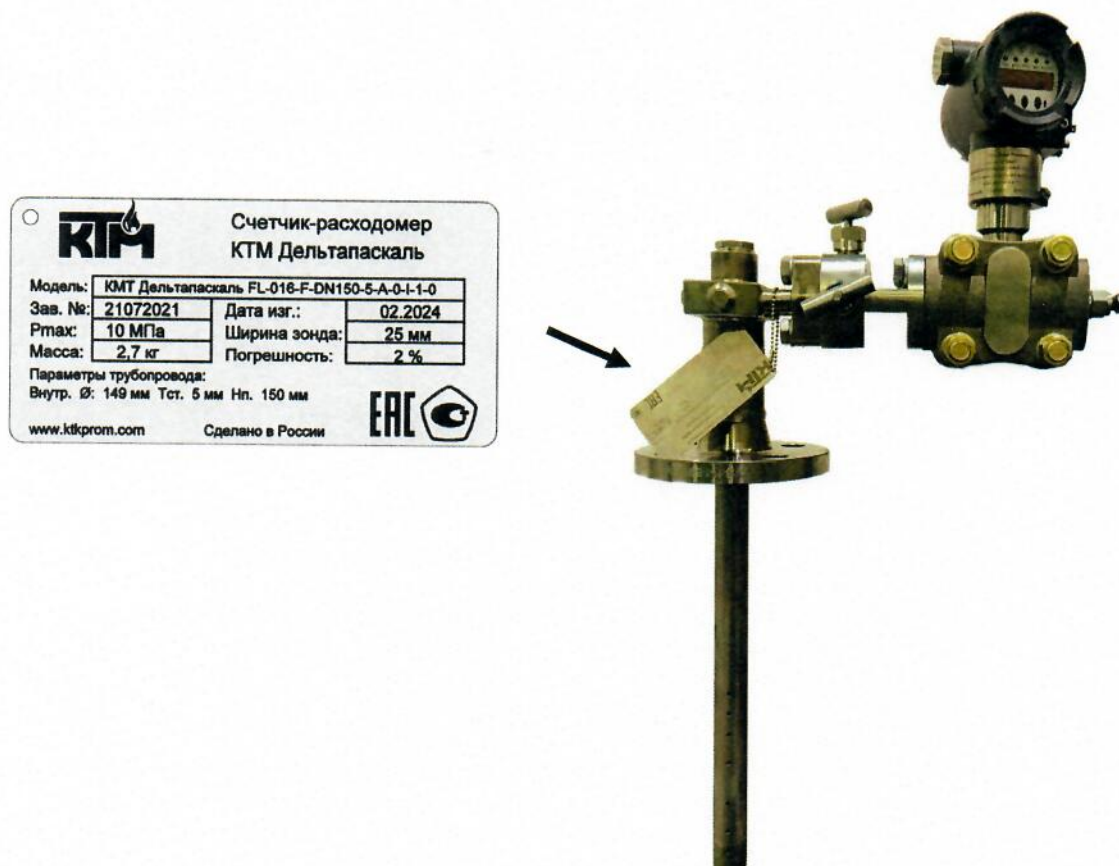
Рисунок 2 – Счётчик-расходомер КТМ Дельтапаскаль без БОИ
